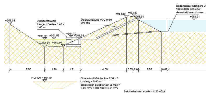
SCHNITT B-B 1:100
